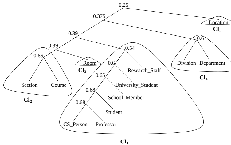
Figura 6. Albero delle affinità: clusters con \sigma = 0.5 .
